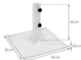
Base metalica cuadrada 50x50x0,8 - 20Kg
