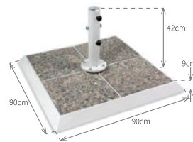
Base metalica con 8 baldosas 90x90x9 - 185Kg
