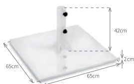
Base metalica cuadrada 65x65x2 - 75Kg
