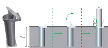
Base para empotrar con tapa abatible
