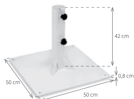
Base metalica cuadrada 50x50x0,8 - 20Kg
