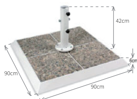
Base metalica con 4 baldosas 90x90x6 - 110Kg
