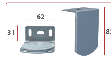
SOPORTE LARGO
