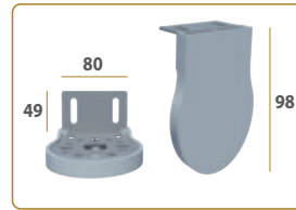
SOPORTE STANDARD
