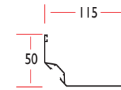
Perfil canal LED
