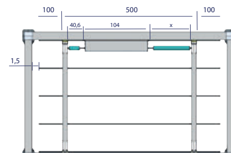
MESURES MAXIMUM : PILIERS À PILIERS
