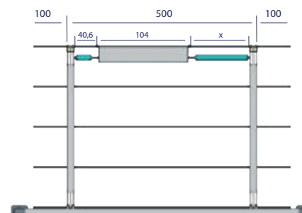
MESURES MAXIMUM : MUR À PILIERS
