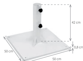
Pied métallique carrée 50x50x0,8 - 20Kg
