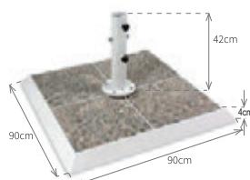
Pied métallique avec 4 tuiles 90x90x4 - 85Kg
