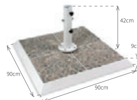
Pied métallique avec 8 tuiles 90x90x9 - 185Kg
