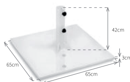
Pied métallique carrée 65x65x3 - 105Kg
