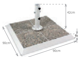
Pied métallique avec 4 tuiles 90x90x6 - 110Kg
