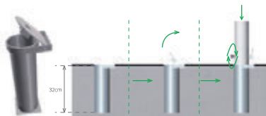
Pied pour encastrer avec bouchon abatible
