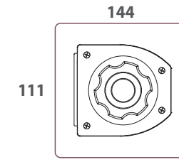
PROFIL COFFRE
